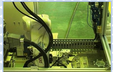
電気小部品自動組立機
