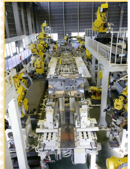
フロントアンダー溶接ライン
