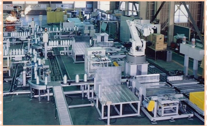
検査梱包ライン
